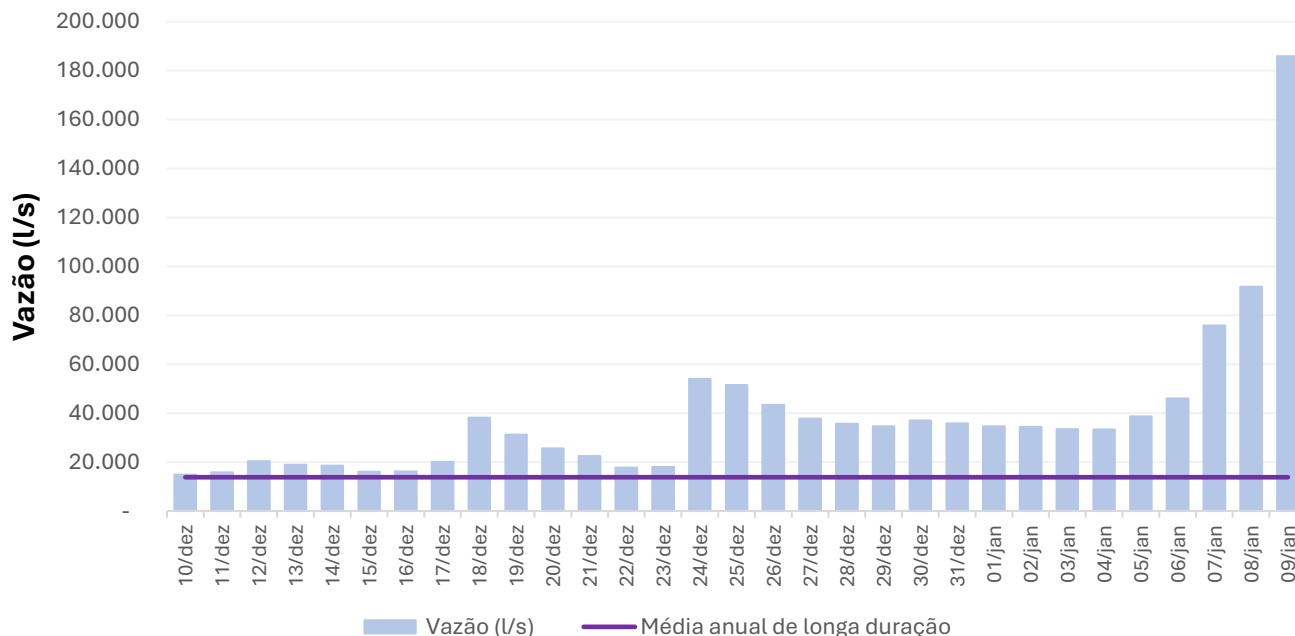
Vazão do Rio Santa Maria da Vitória nos últimos 30 dias
