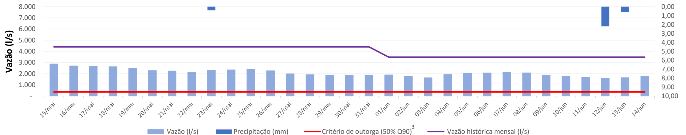
Histórico de vazão e precipitação nos últimos 30 dias
